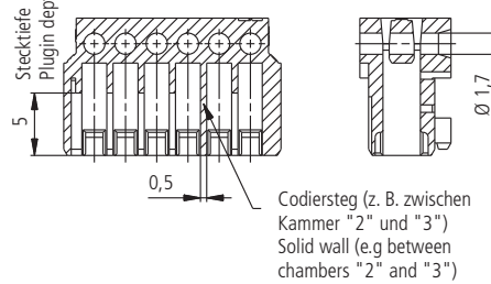
Darstellung ohne Kontakte Designation without contacts
