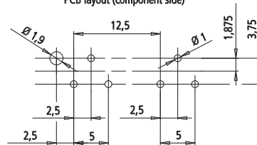
Lochbild (Bauteilseite) PCB layout (component side)
