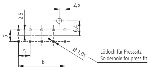
Lochbild (Bestückungsseite) Hole pattern (component side)
