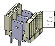
Farbkennzeichnungsbereich bei versilberten Kontakten colour coding area when silvered contacts (nach / according WN 30.70 Bereich / area "D")
