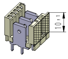
Farbkennzeichnungsbereich bei versilberten Kontakten colour coding area when silvered contacts (nach / according WN 30.70 Bereich / area "D")
