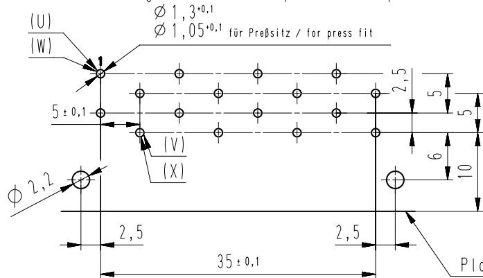
Lochbild (Bestückungsseite) / hole pattern (component side)
