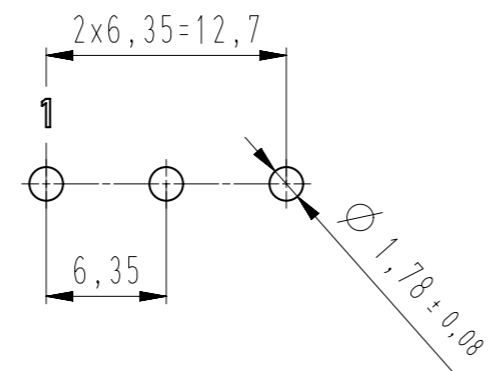
Lochbild von der Bestückungsseite hole pattern by the component side
